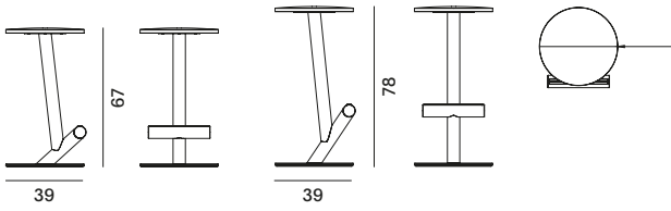
versione girevole H67,8
